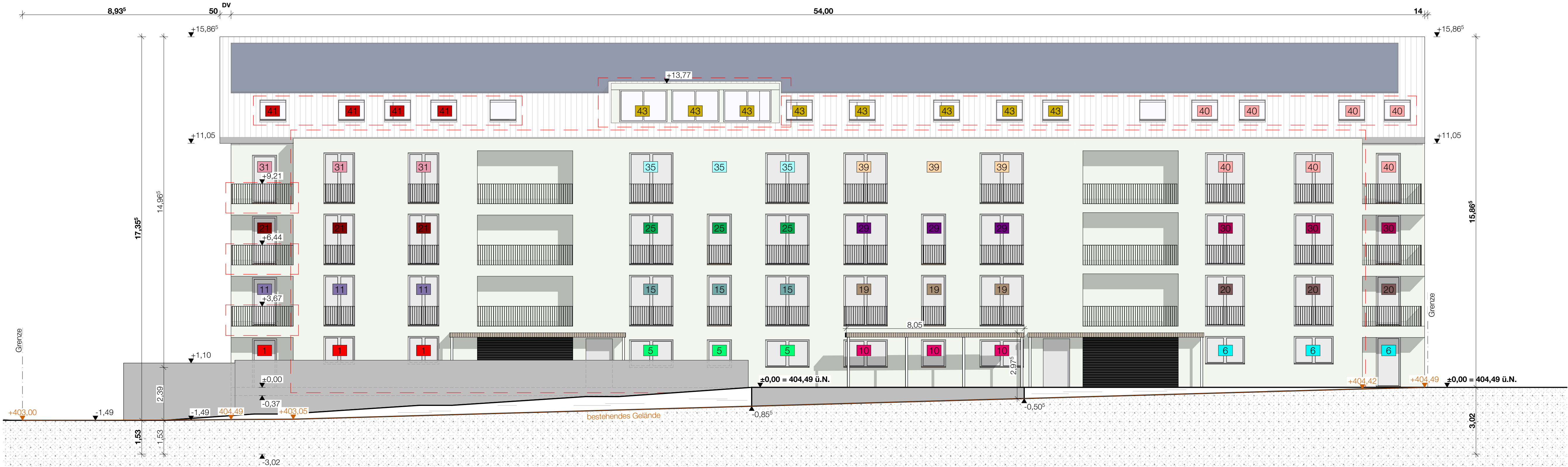
Ansicht Süd-Ost
