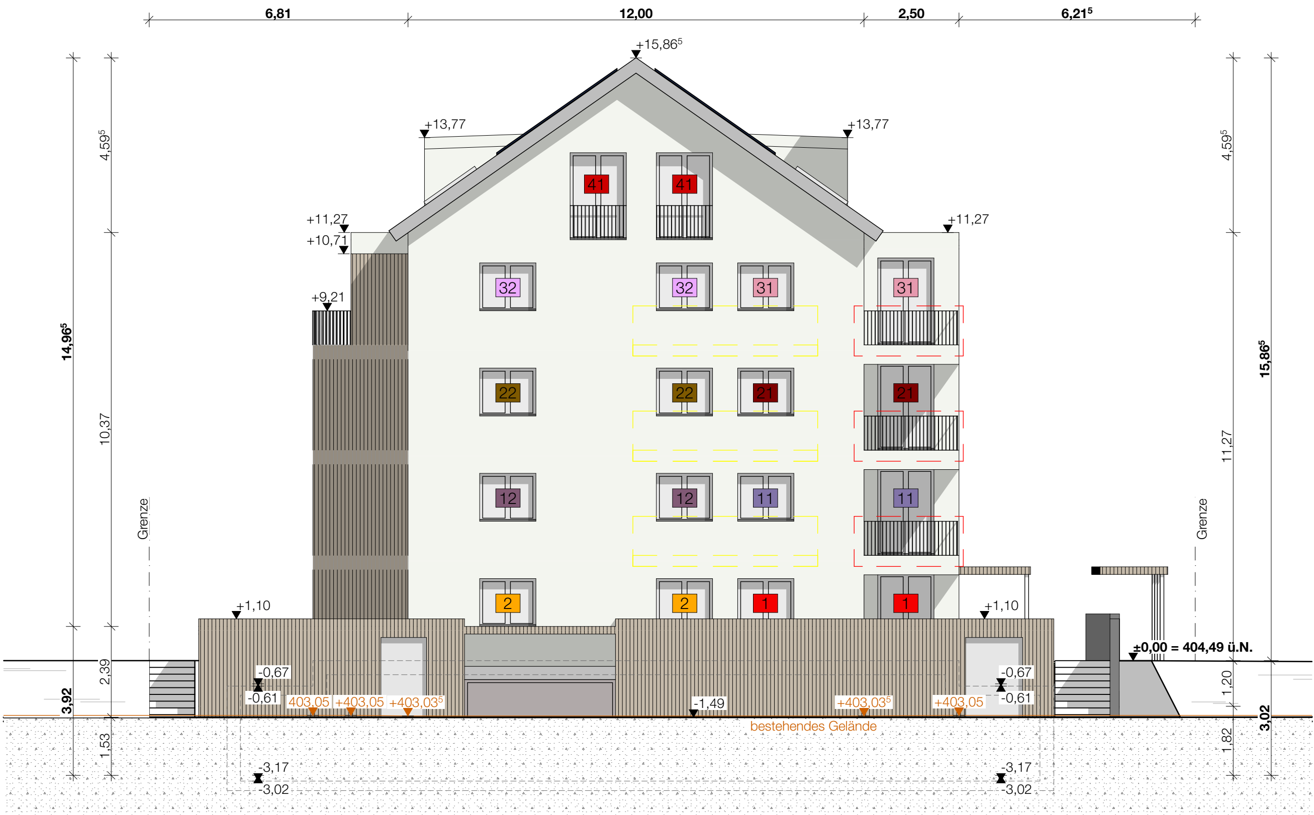
Ansicht Süd-West
