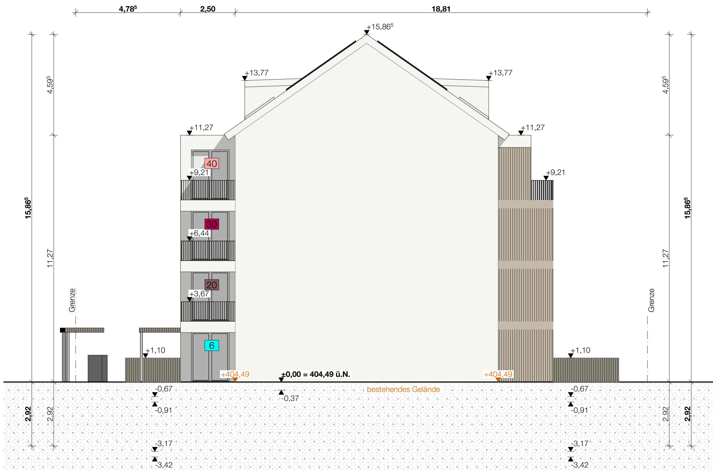
Ansicht Nord-Ost
